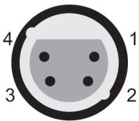
XLR-4F
